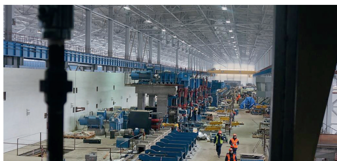
Монтаж крупногабаритного промышленного производственного оборудования к бетонным фундаментам при проведении реконструкции (сквозной монтаж после установки конструкций в проектное положение)
