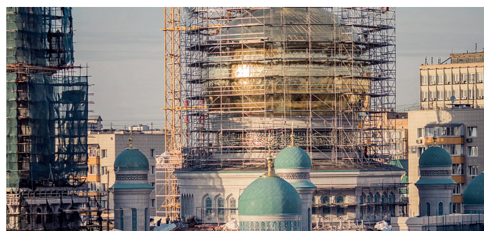
Крепление наружной и внутренней облицовки: 2500 тонн сложных декоративных изделий из гранита (Московская Соборная мечеть, г. Москва, 2015 г.)
