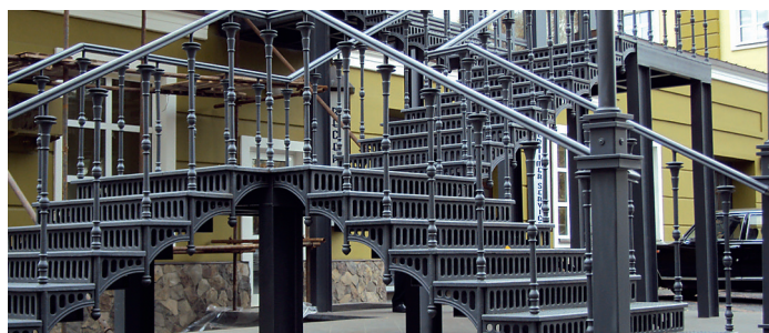
Крепление массивных литых элементов чугунных конструкций лестничного марша, выполненного по индивидуальному проекту (Музей техники Вадима Задорожного, Красногорский район Московской области, 2007 г.)
