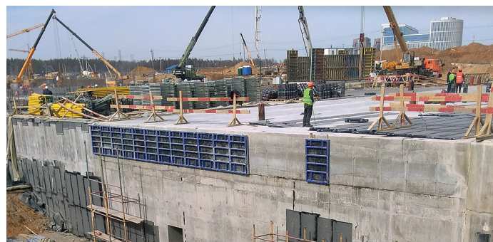
Организация арматурных выпусков при строительстве многоуровневой развязки и тоннеля под Калужским шоссе в районе ТПУ «Столбово» (Москва, 2018 г.)
